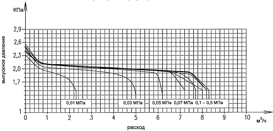
Характеристика регуляции RTP 6-М...-
